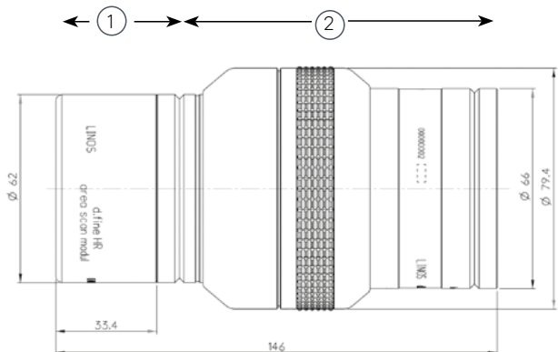
① d.fine HR area scan module ② d.fine HR 2.4/128 3.33x
